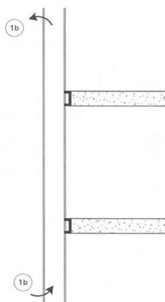
Façade double paroi non segmentée (ventilation multi-étages)
