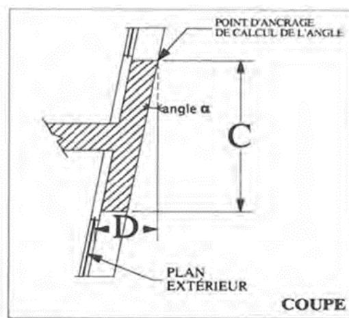
Figure 2.4.2 : Façade inclinée vers l'extérieur
