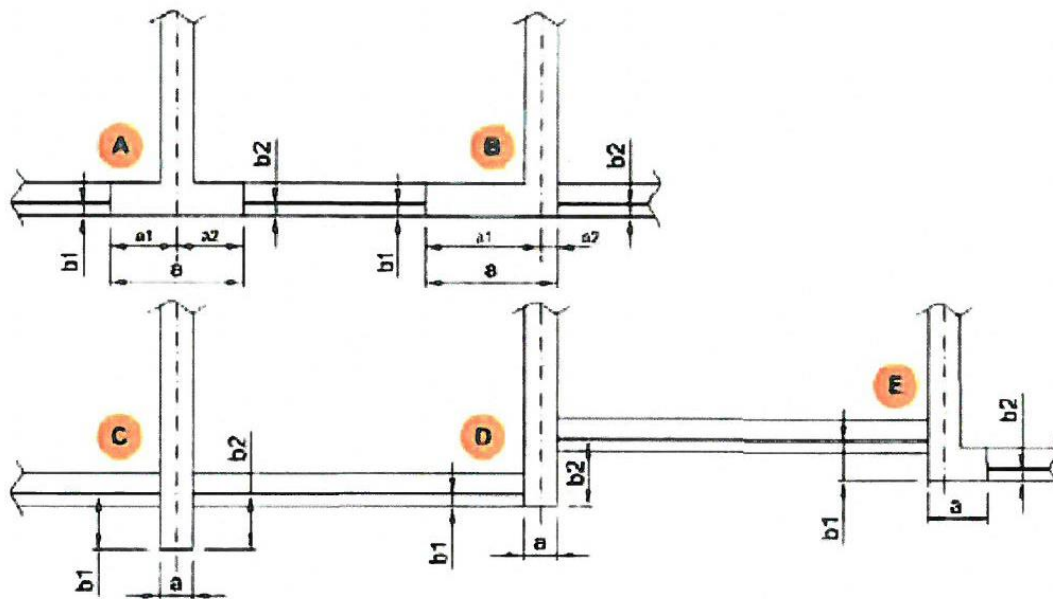
Figure 5 : Option 1 (coupes horizontales)
