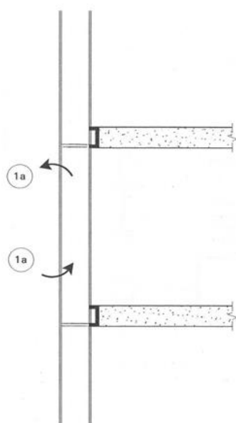
Façade double paroi segmentée (ventilation par étage)
