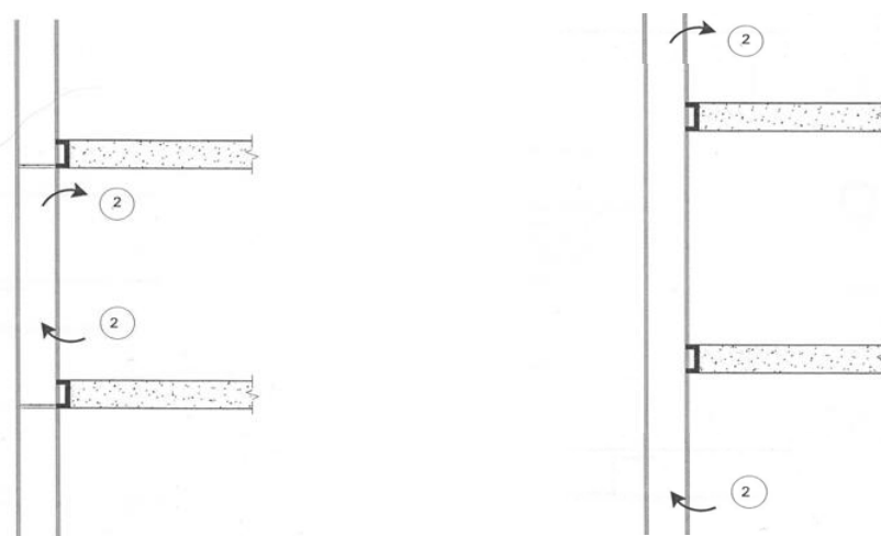
Façade double paroi segmentée (ventilation par étage)
